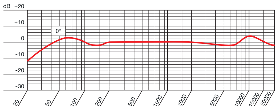
Frequenzkurve
