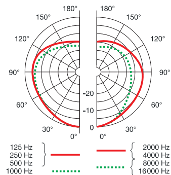
Polardiagramm
